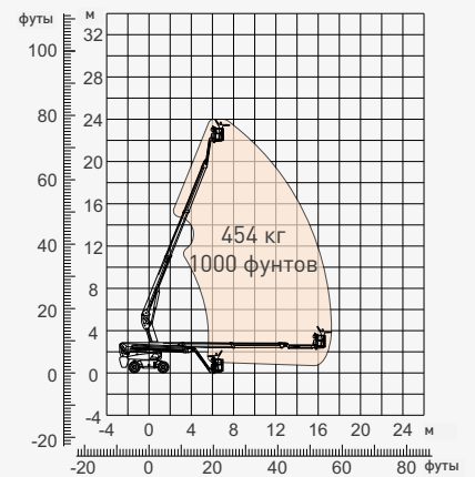
Диапазон перемещения
